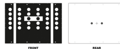
Placa de calibração para VW + MB Ref. n.º WW01000670
