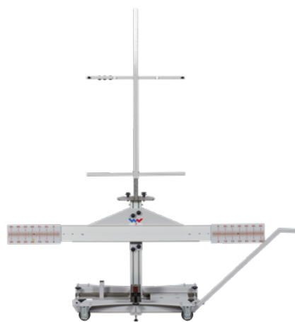
Suporte universal para placas de calibração (alvos)* Ref. n.º WW01000661
