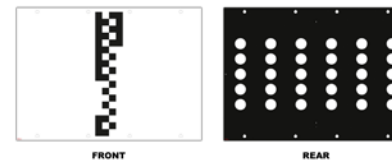
Kalibrálótábla FCA + Alfa Cikksz. WW01000672
